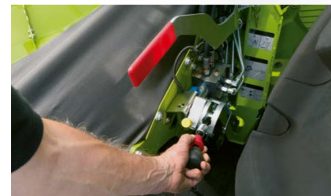
Adaptación en tres niveles del régimen de revoluciones de los cilindros de alimentación para un flujo de material óptimo.
