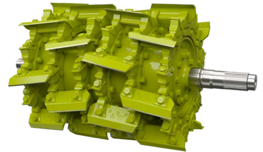
V-FLEX avec demi-couteaux pour doubler la longueur de coupe avec un flux de récolte symétrique
