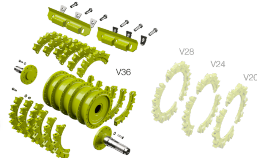
Un corps de base pour un montage flexible, plusieurs configurations de couteaux et des segments circulaires ultra-résistants à l'usure
