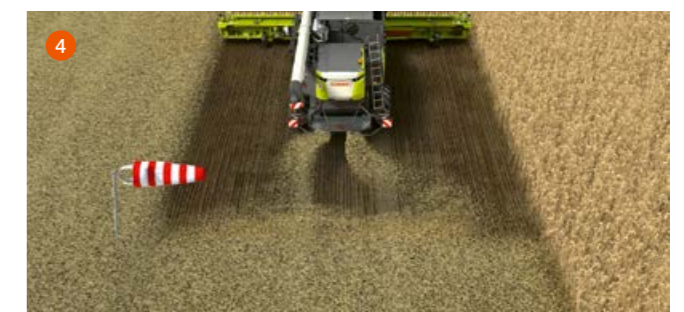
3 Датчики в задней части машины определяют интенсивность бокового ветра.
