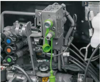
Le freinage hydraulique de remorque double ligne assure une grande polyvalence au transport.
