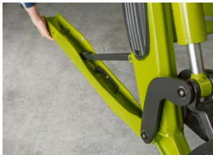
Los apoyos se pliegan fácilmente debajo del montante, y, por lo tanto, no interrumpen la visión del cargador frontal.
