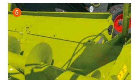
Die zusätzliche Rückwandlerhöhung (5) verhindert das Entstehen von Spritzverlusten bei Raps.
