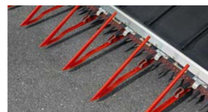
Podnośniki łań można wymieniać szybko i bez użycia narzędzi.
