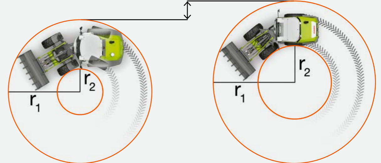
TORION SINUS mit gelenkter Hinterachse
