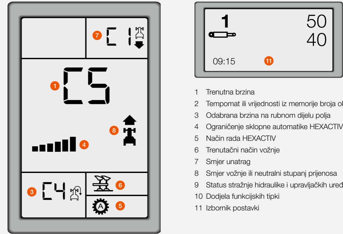
Zaslon CIS na nadzornoj ploči i zaslonu mjenjača na A-stupu.
